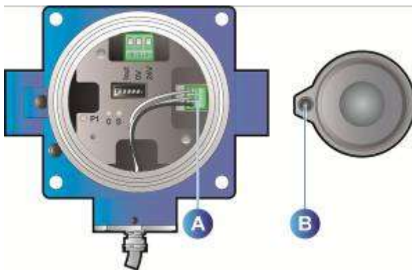
Рис 17: OLCT 100HT – особые элементы замены высокотемпературного датчика
