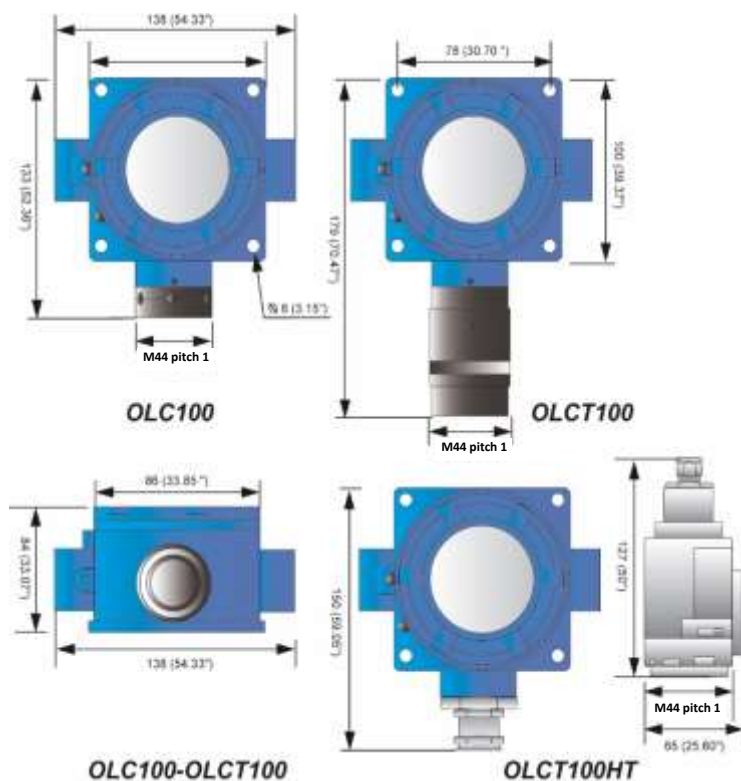
Рис 18: геометрические характеристики детекторов
