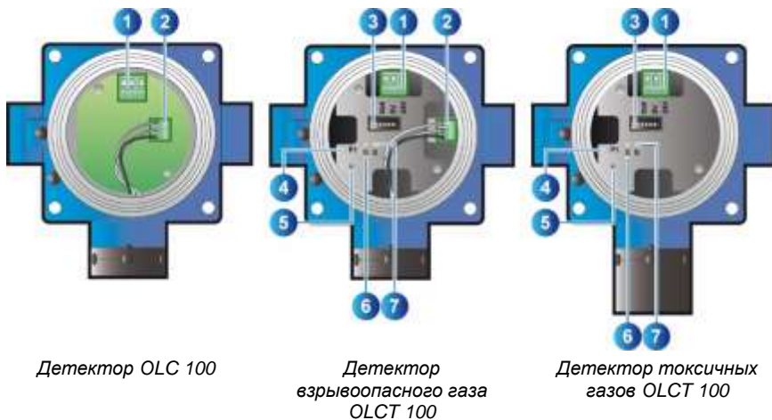
Рис 2 : вид детекторов изнутри
