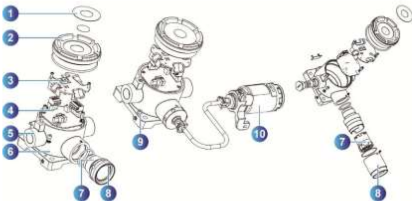
Рис 1 :компоненты детектора OLCT 100
